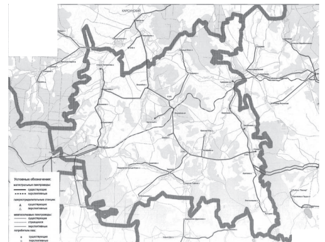
Схема газоснабжения и газификации Вешкаймского района Ульяновской области
