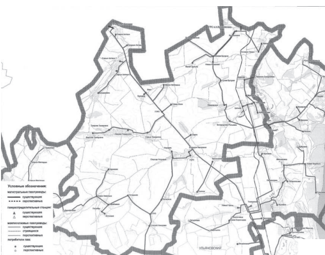
Схема газоснабжения и газификации Цильнинского района Ульяновской области
