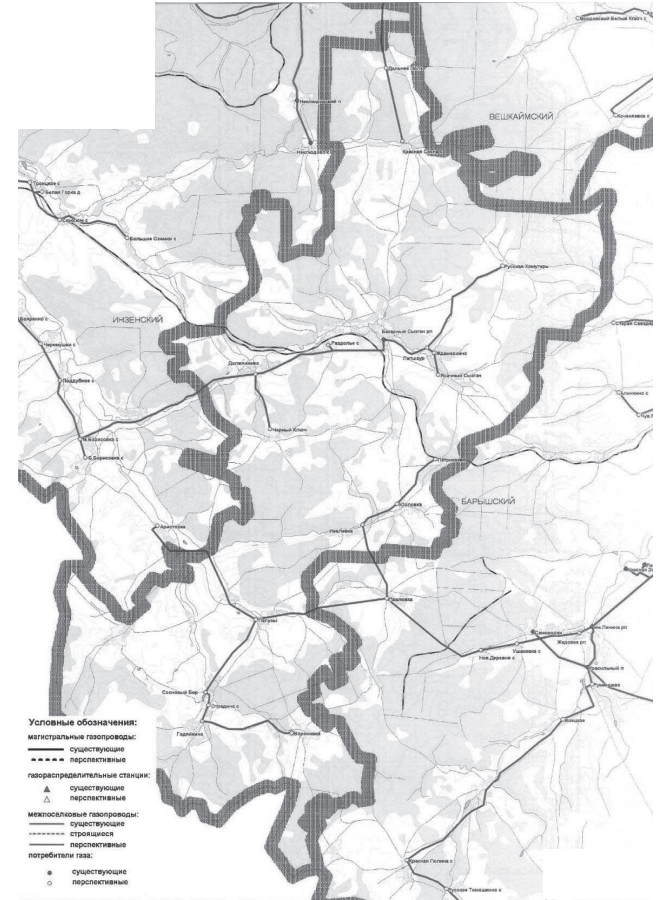
Схема газоснабжения и газификации Базарносызганского района Ульяновской области
